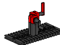
Kegelradgetriebe / Bevel gear / Engrenage à pignon conique / Conische tandwieloverbrenging / Engranaje de ruedas cónicas / Engrenagem cônica
